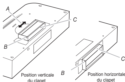
A. Ajustement latéral jusqu'à 1" (2,5 cm) B. Pivot C. Module connecteur/clapet
